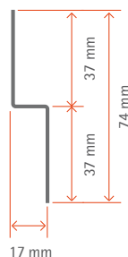
Z-Profil
